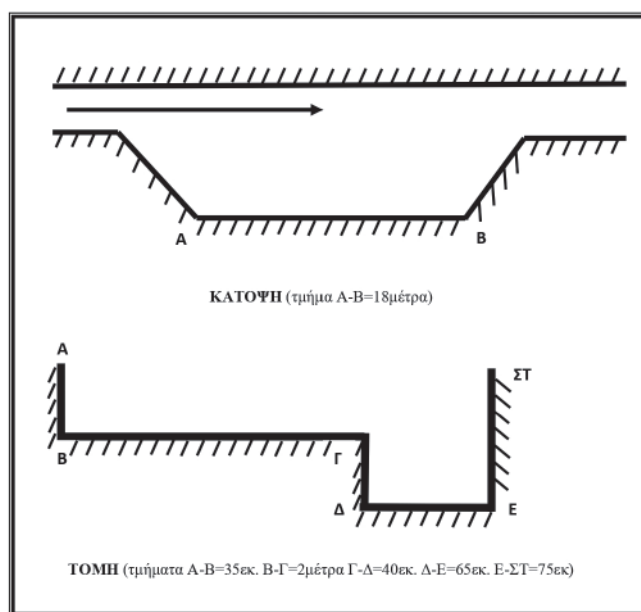
Εικ. 3. Κάτοψη και τομή τσιμεντένιας κατασκευής στην τοποθεσία Ταμπάχανα, όπως είναι σήμερα (2021).
