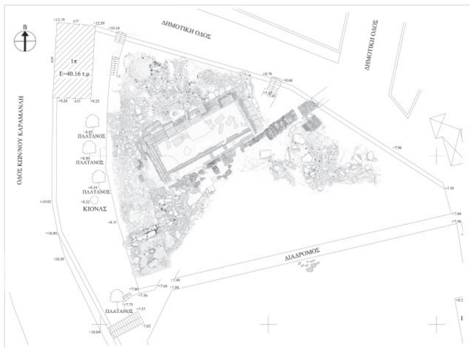
Εικ. 16. Υπέρεια Κρήνη Φερών. Κάτοψη του κρηναίου οικοδομήματος. Κλίμακα 1:50.
