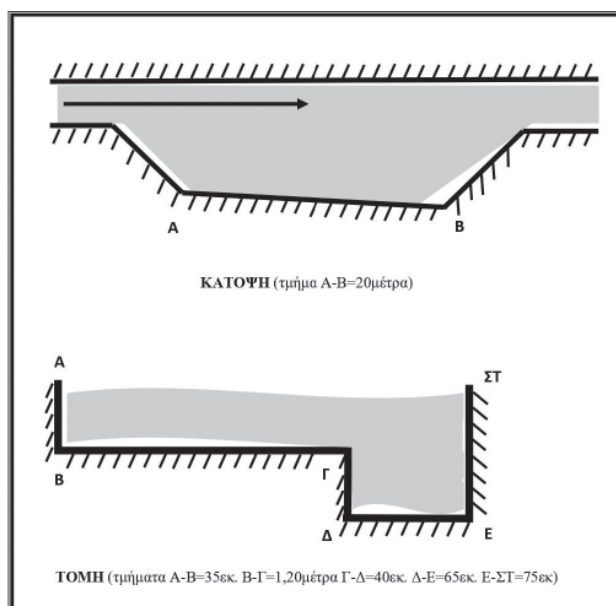
Εικ. 17. Κάτοψη και τομή τσιμεντένιας κατασκευής στην πορεία του κεντρικού αυλακιού προς Μύλο Μπαλαμώτη, όπως είναι σήμερα (2021).
